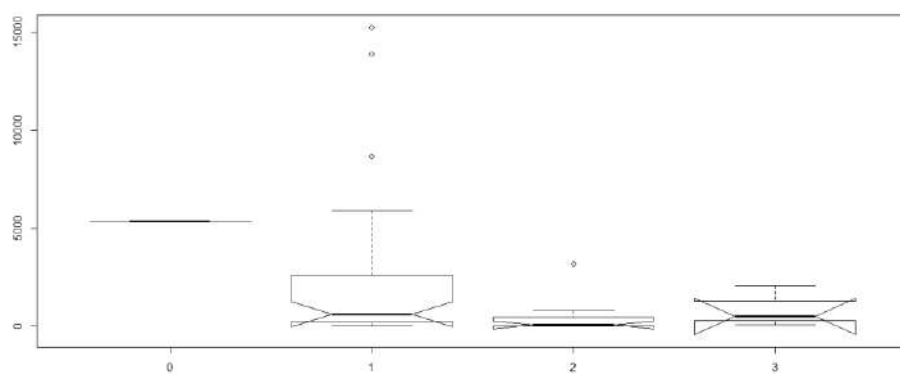
Figure 65 : Nombre moyen de captures en civelles en 2007 en fonction des indices de débits
