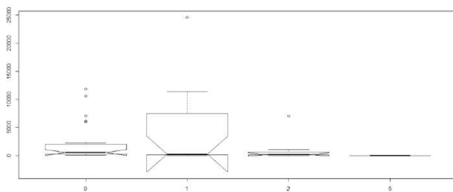
Figure 64 : Nombre moyen de captures en civelles en 2006 en fonction des indices de débits
