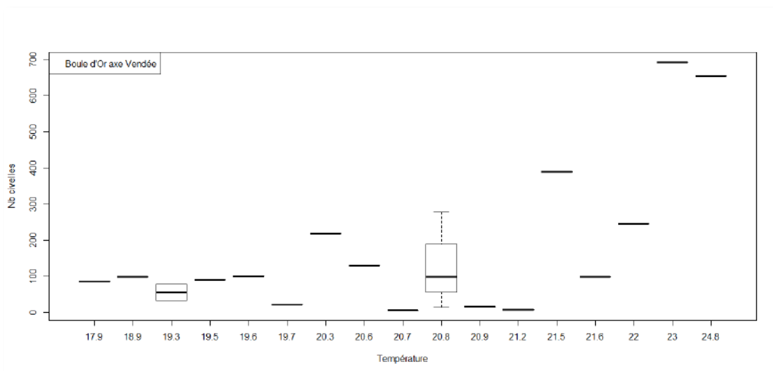
Figure 11 : Nombre de civalles recensées à Boule d'Or axe Vendée en fonction de la température
