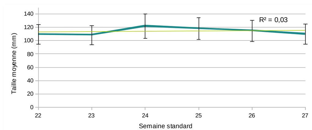
Figure 44 : Evolution saisonnière de la taille moyenne des civelles à Boisse en 2012
