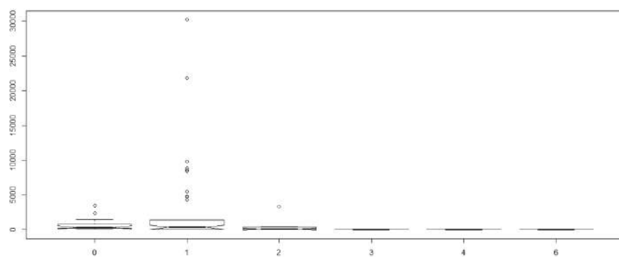
Figure 66 : Nombre moyen de captures en civelles en 2008 en fonction des indices de débits
