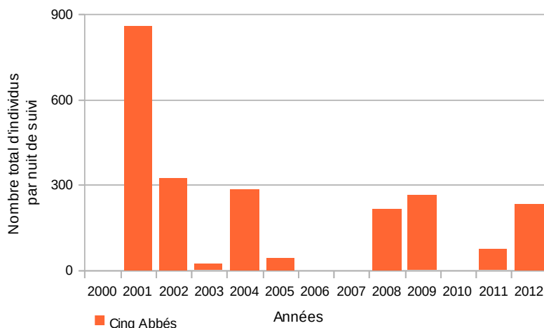
Figure 25 : Résultats des captures de civelles par nuit de suivi aux Cinq Abbés entre 2000 et 2012
