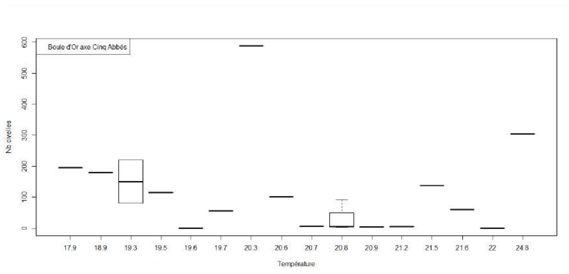
Figure 12 : Nombre de civalles recensées à Boule d'Or axe Cinq Abbés en fonction de la température
