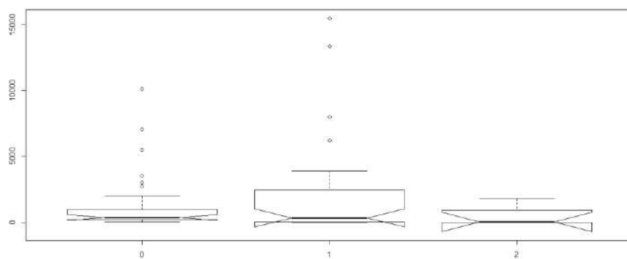
Figure 63 : Nombre moyen de captures en civelles en 2005 en fonction des indices de débits
