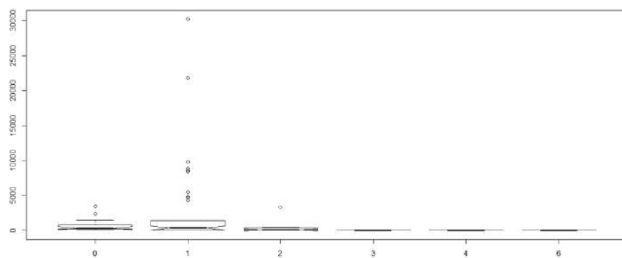
Figure 68 : Nombre moyen de captures en civelles en 2010 en fonction des indices de débits
