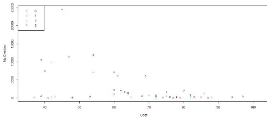
Figure 51 : Nombre de civelles capturées par nuit de suivi en 2006 en fonction des coefficients de marée et des indices de débits
