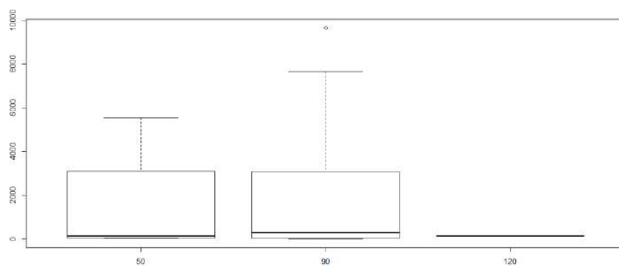
Figure 81 : Nombre moyen de captures en civelles en 2010 en fonction des coefficients de marée
