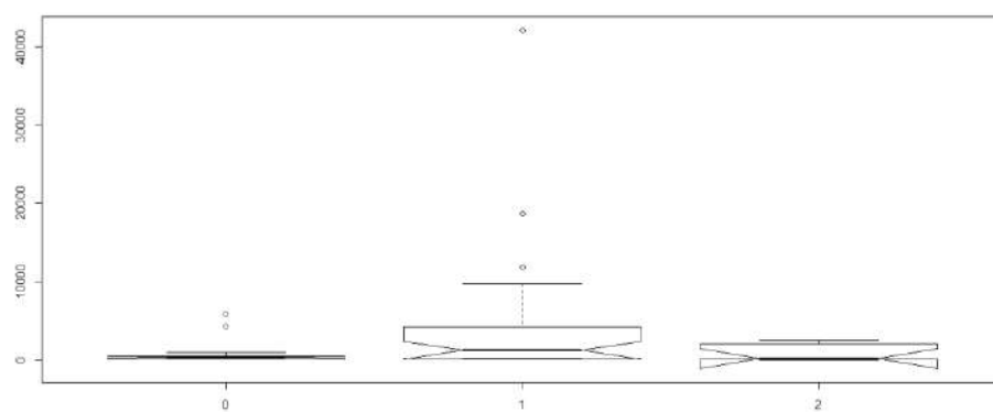
Figure 67 : Nombre moyen de captures en civelles en 2009 en fonction des indices de débits
