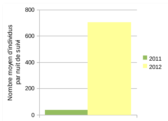
Figure 40 : Bilan des captures de civelles à Boisse en 2011 et 2012
