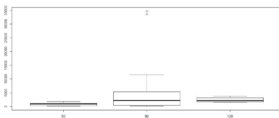
Figure 71 : Nombre moyen de captures en civelles en 2000 en fonction des coefficients de marée
