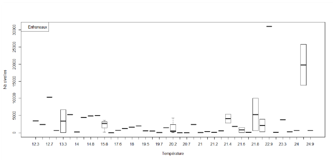
Figure 6 : Nombre de civelles recensées aux Enfreneaux en fonction de la température
