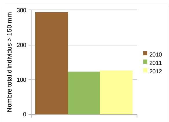
Figure 30 : Bilan des captures de gros individus à Boule d'Or Vendée de 2010 à 2012
